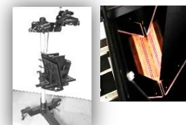
開発品：貴重洋書用 30度見開きデジタル撮影システム
